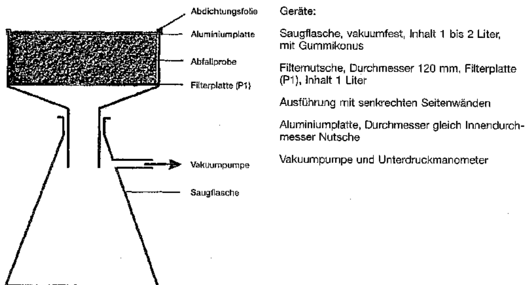
Bild 1: Apparatur zur Einstellung des Wassergehaltes
